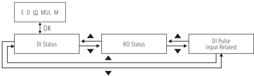
Fig. 3-13 IO Display
