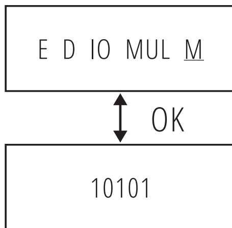
Fig. 3-23 Shortcut Code
