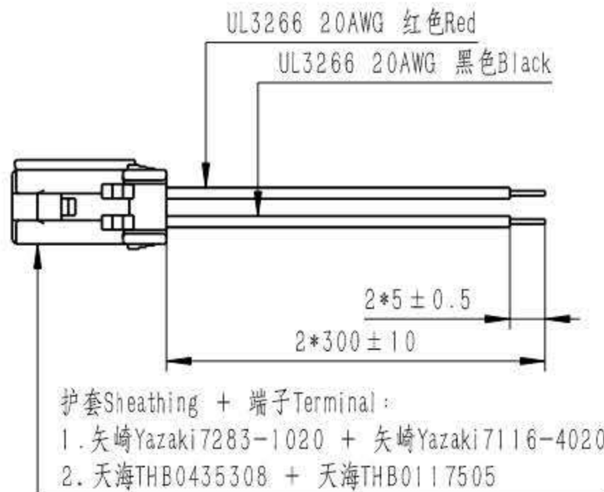
线圈连接器(选配) Coil Connector(Optional)
