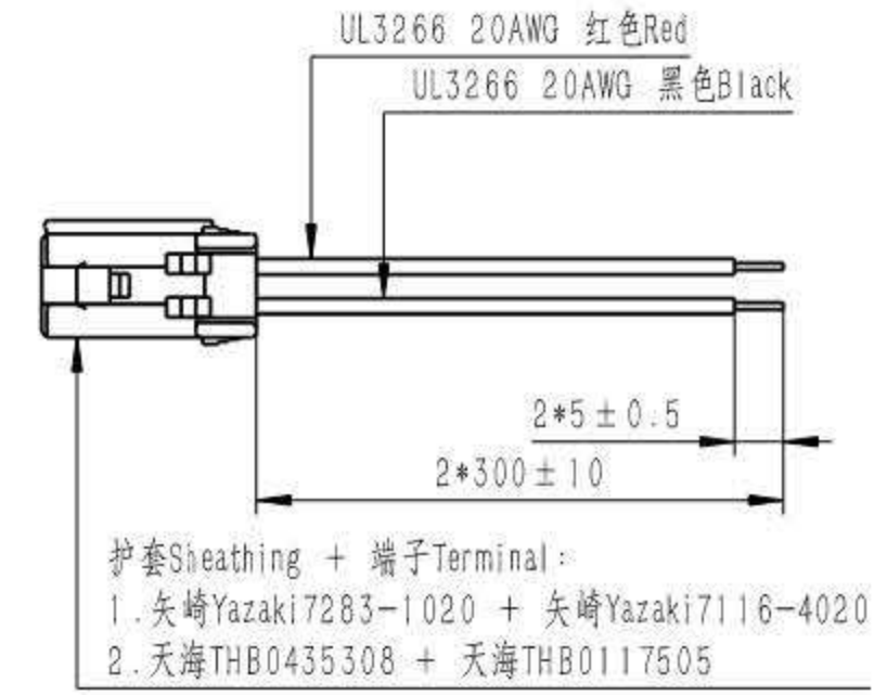
线圈连接器(选配) Coil Connector(Optional)
