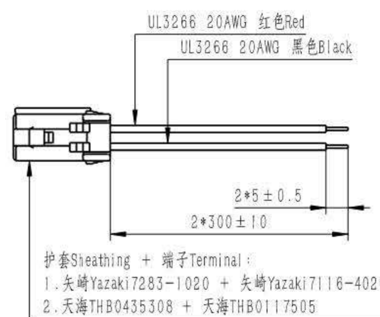
线圈连接器(选配) Coil Connector(Optional)
